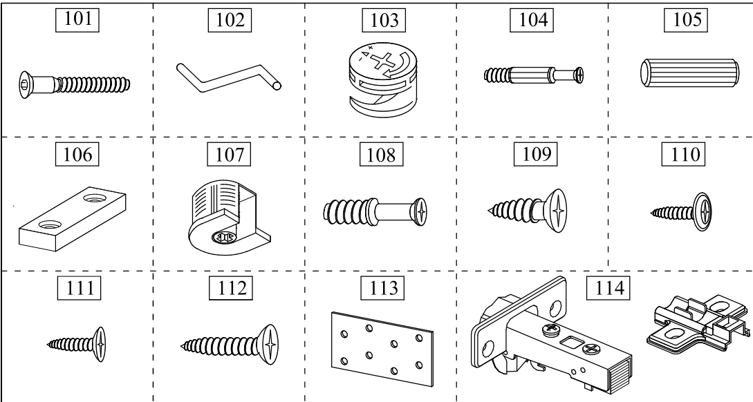
Ведомость фурнитуры
